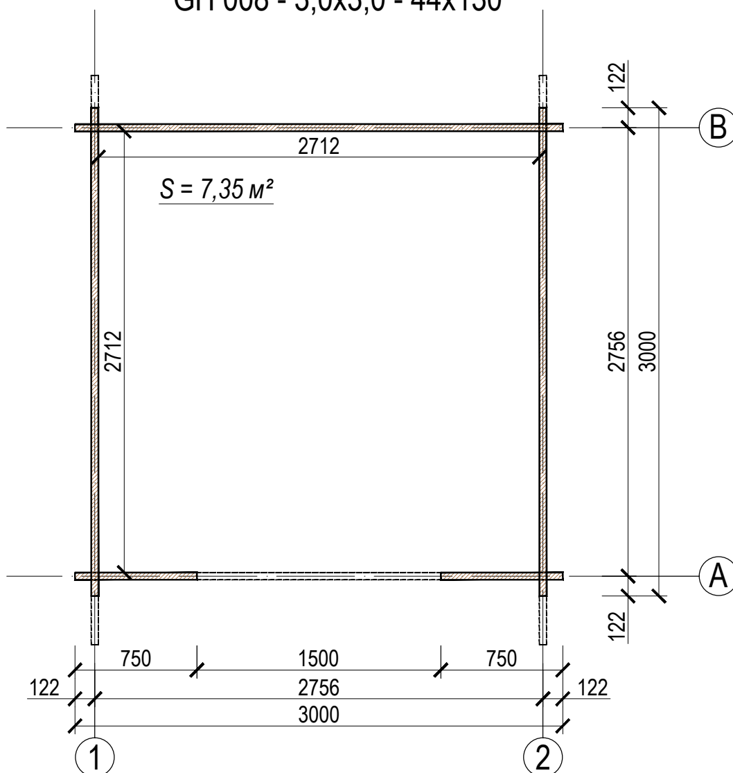
План в осях 1/2 - А/В ГН 008 - 3,0х3,0 - 44х130
