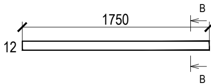
Верхняя ветрозащитная планка
